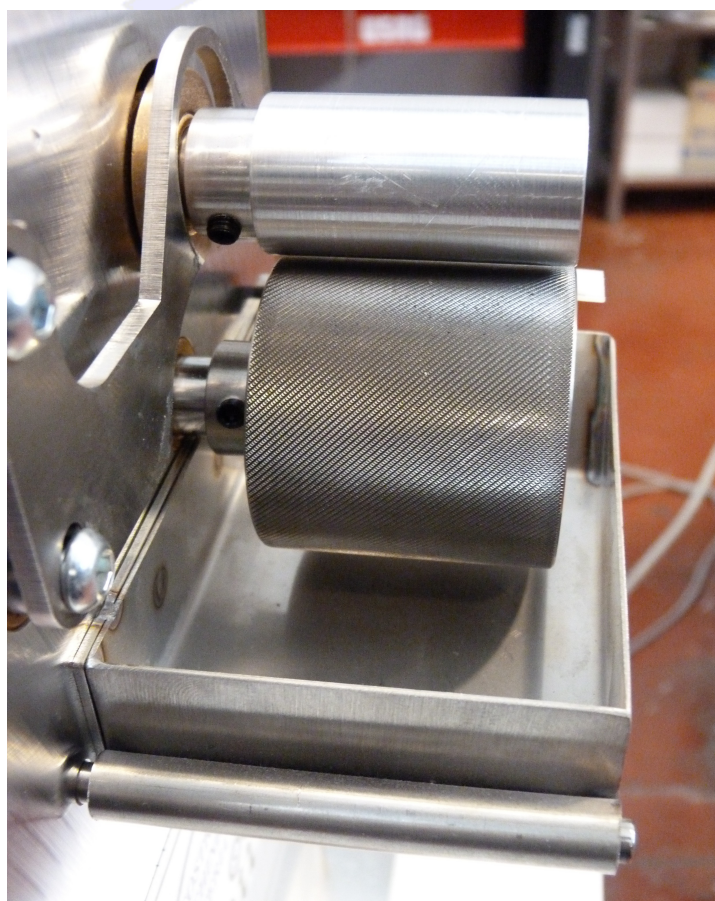
MODELLO 177-VR XL con rulli da 45 mm
