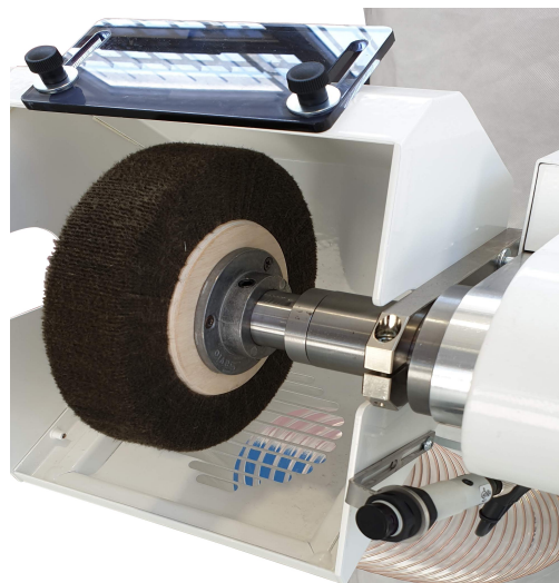
Versione 750-VRAVP TOUCH PLUS con Aspiratore var. e sensori di prossimità
